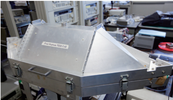
4-Septum TEM Cell
