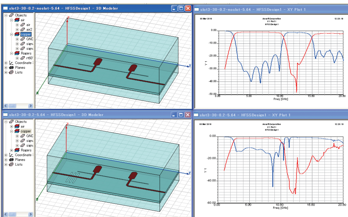
グラントの欠落を利用する広帯域マイクロ波フィルタ
