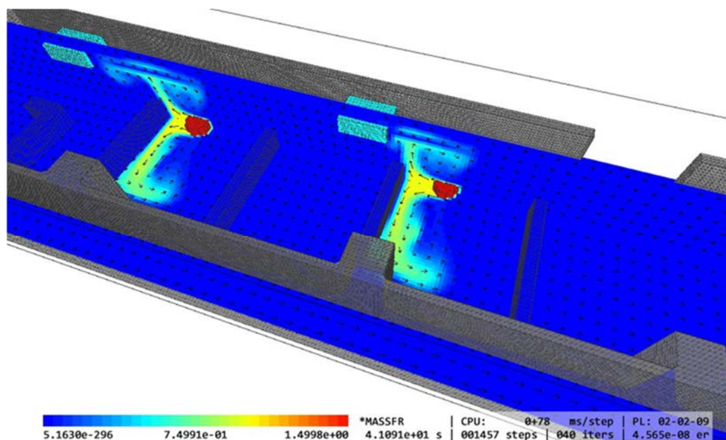
熱流体シミュレーションによる解析結果 (感染者の呼気がパーティション区画内に広まる様子)
